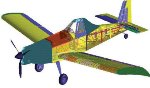
Şekil 3- ZIU CAD modeli.
